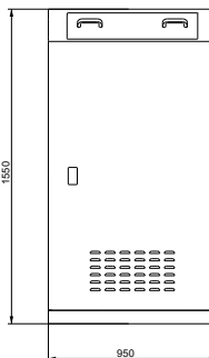
Ön Görünüş
