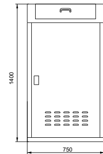
Ön Görünüş
