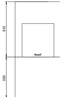
Üst Görünüş
