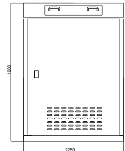
Ön Görünüş
