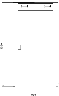
Ön Görünüş
