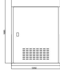
Ön Görünüş
