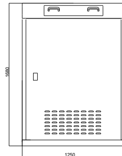
Ön Görünüş
